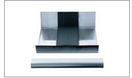
Expansie-element compleet met separaat kraalstuk, voor bak- en mastgoot
